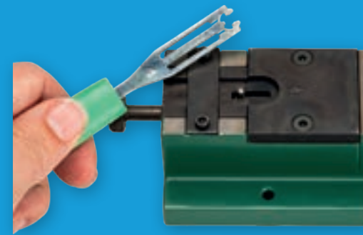
Montagegreifer für DIN 6799 Dispenser Base for DIN 6799
